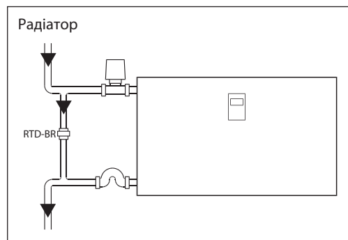
RTD-BR на замикальній ділянці стояку однотрубної системи опалення.
