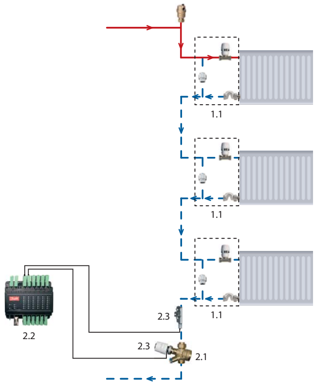
Приклад підбору обв'язки опалювального приладу при русі теплоносія в стояку «зверху вниз»
