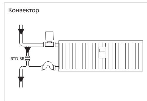
RTD-BR на замикальній ділянці стояку однотрубної системи опалення.
