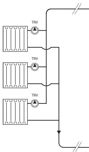
Рис. 21. Клапани терморегуляторів з функцією автоматичного регулювання перепаду тиску та обмеження витрати на опалювальних приладах двотрубно́ї системи опалення із змішаною розводкою магістральних трубопроводів
