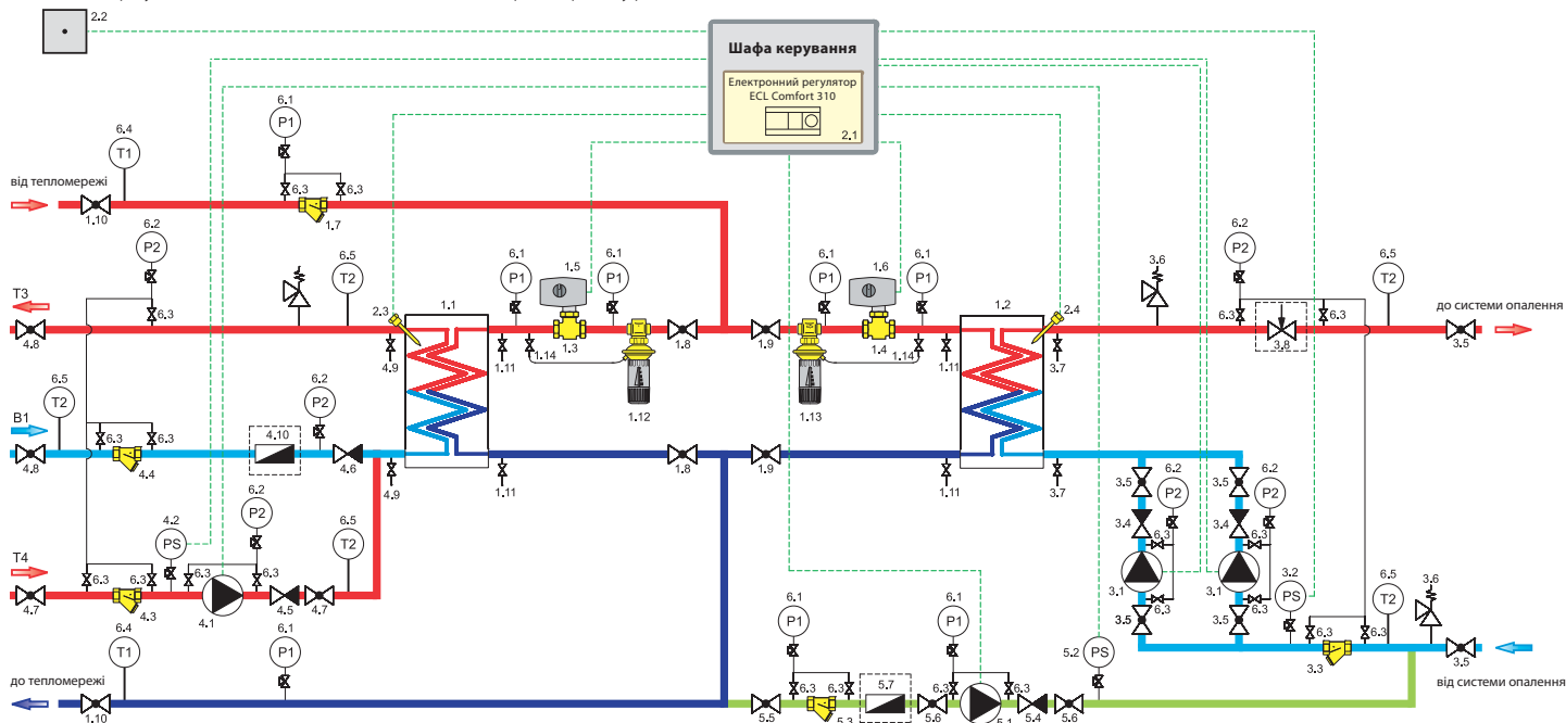
Рис. 26. Принципова схема двоконтурного ІТП: система опалення із незалежною схемою підключення та система ГВП будинку
