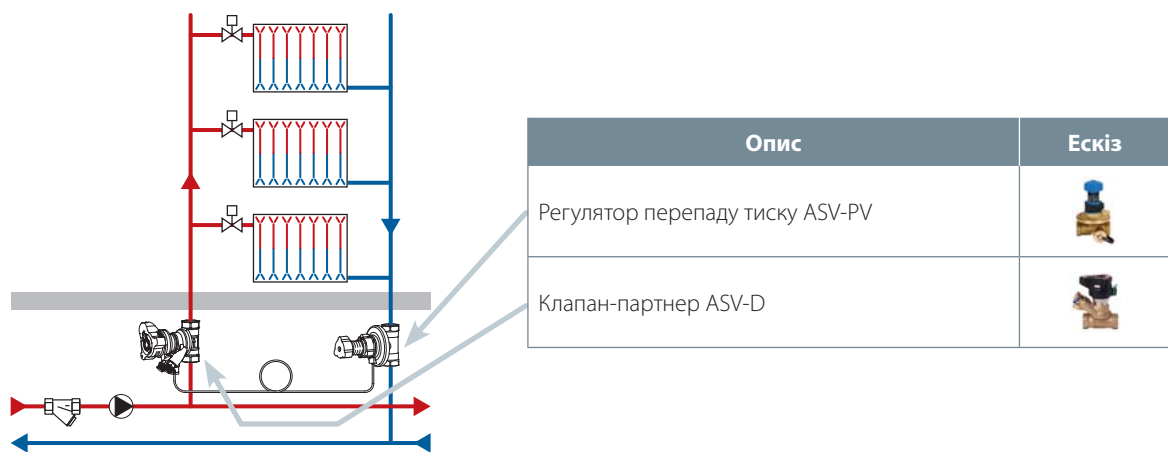
Рис. 9. Стабілізація перепаду тиску в стояку вертикальної двотрубної системи опалення зі змінним гідралічним режимом
