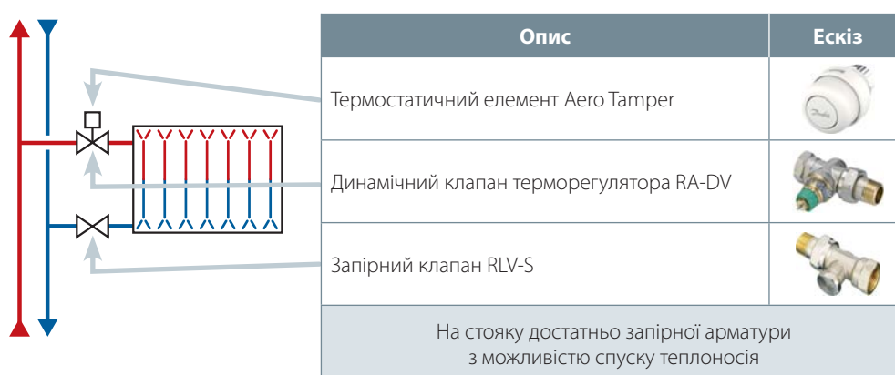
Рис. 6. Приклад комплектації вузла обв'язки опалювального приладу в двотрубній системі опалення з динамічним клапаном терморегулятора
