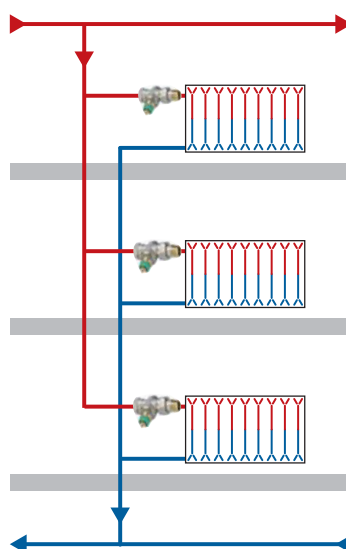
Рис. 7. Клапани терморегуляторів із функцією автоматичного регулювання перепаду тиску та обмеження витрати на опалювальних приладах двотрубною системою опалення зі змішаною розводкою магістральних трубопроводів
