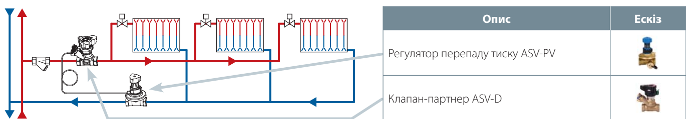
Рис. 10. Стабілізація перепаду тиску в приладовій вітці горизонтальної двотрубної системи опалення зі змінним гідралічним режимом
