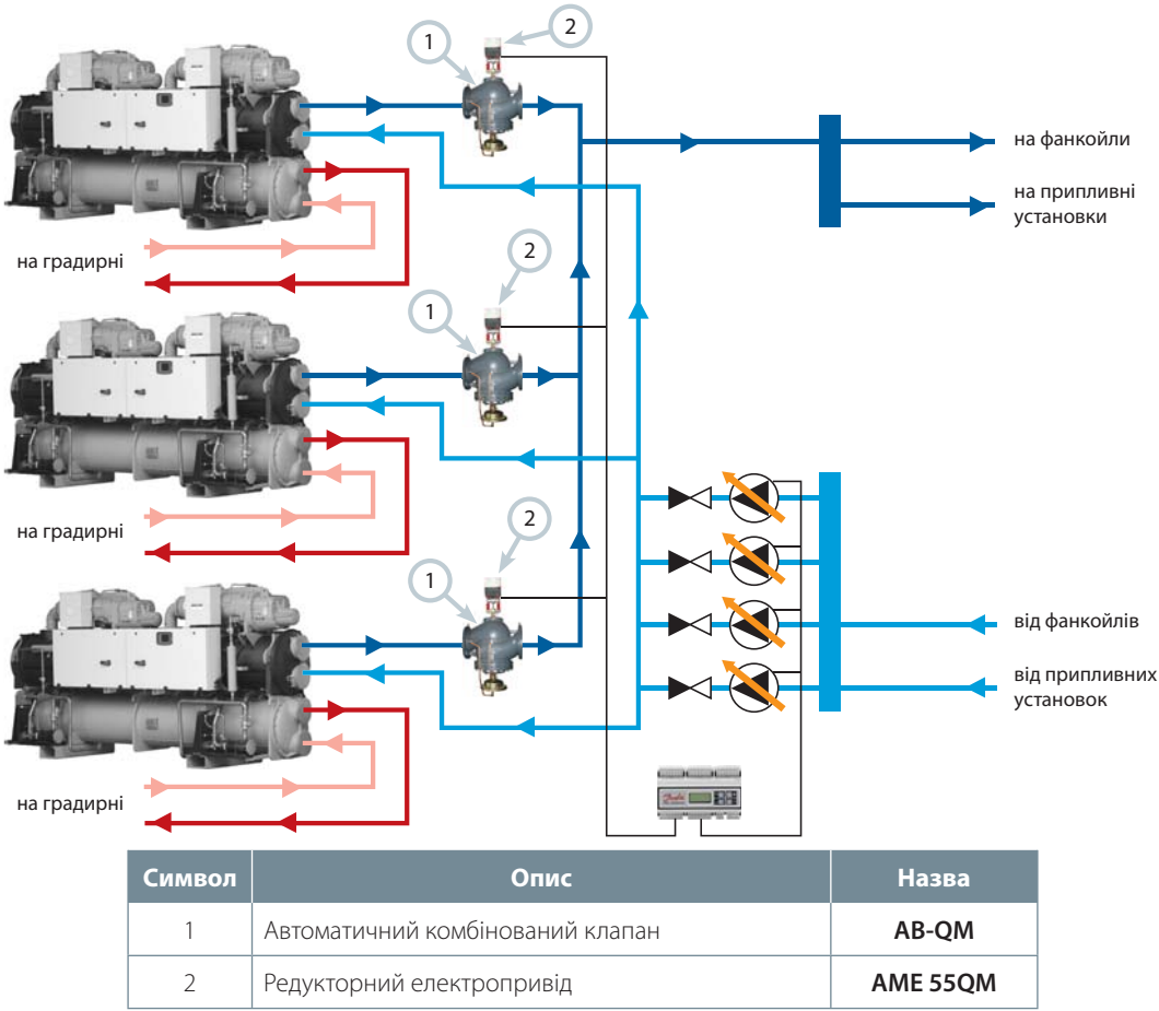
Рис. 20. Обв'язка чиллерів, що працюють в змінному гідравлічному режимі
