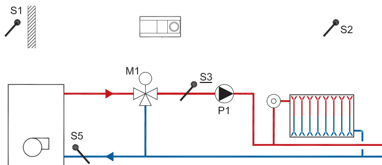
Рис. 2. Один із прикладів вузла регулювання при приєднанні до індивідуального джерела
