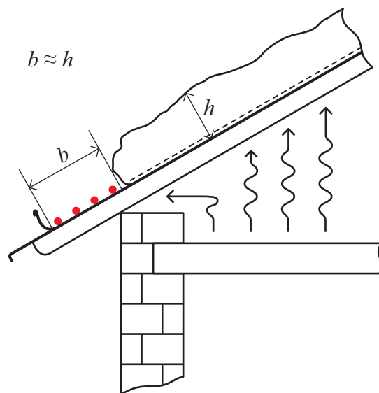
Скатний дах, карниз, вид збоку
