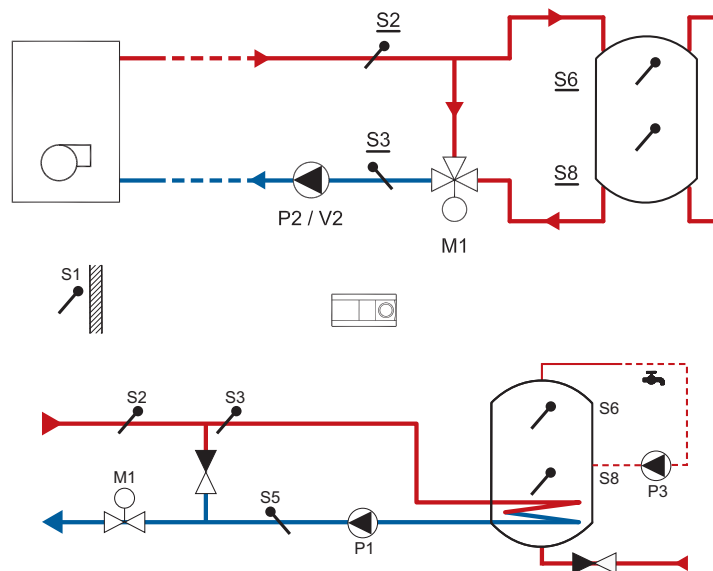
Рис. 3. Приклади схем з баками-акумуляторами
