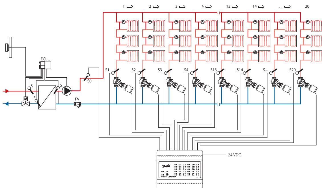
Рис. 13. Обмеження максимальної витрати з регулюванням температури теплоносія на виході стояків у однотрубно́ї системи зі змінним гідравлічним режимом
