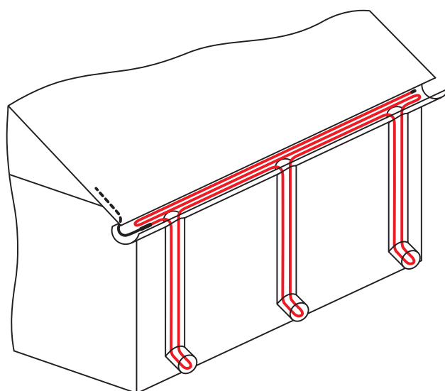
Скатний дах, підвісний жолоб
