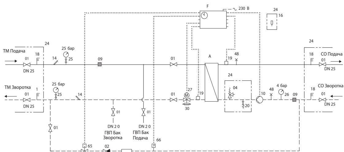
Рис. 2. Принципова схема малого теплового пункту
