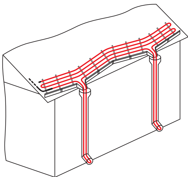
Скатний дах, прикарнизний жолоб
